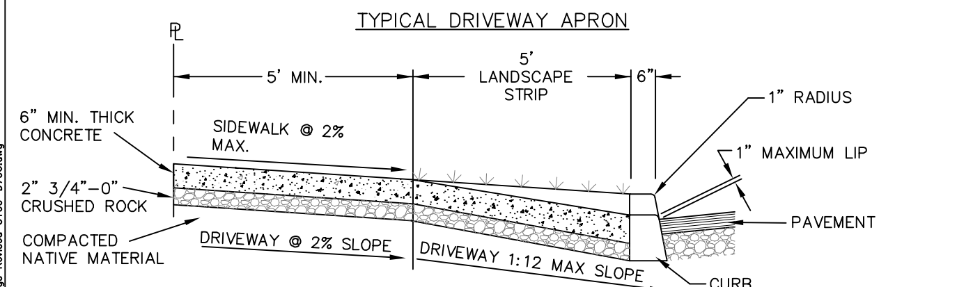
SECTION A-A
